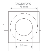
Ghiera orientabile, grigio satinato / Adjustable frame, satin nickel
