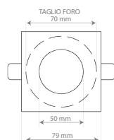
Ghiera fissa, bianco lucido / Fixed frame, glossy white
