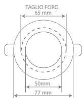
Ghiera fissa, ramato / Fixed frame, red/bronze
