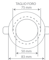
Ghiera orientabile, ramato / Adjustable frame, red/bronze
