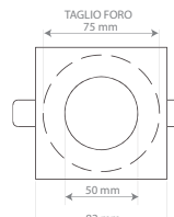
Ghiera orientabile, bianco lucido / Adjustable frame, glossy white
