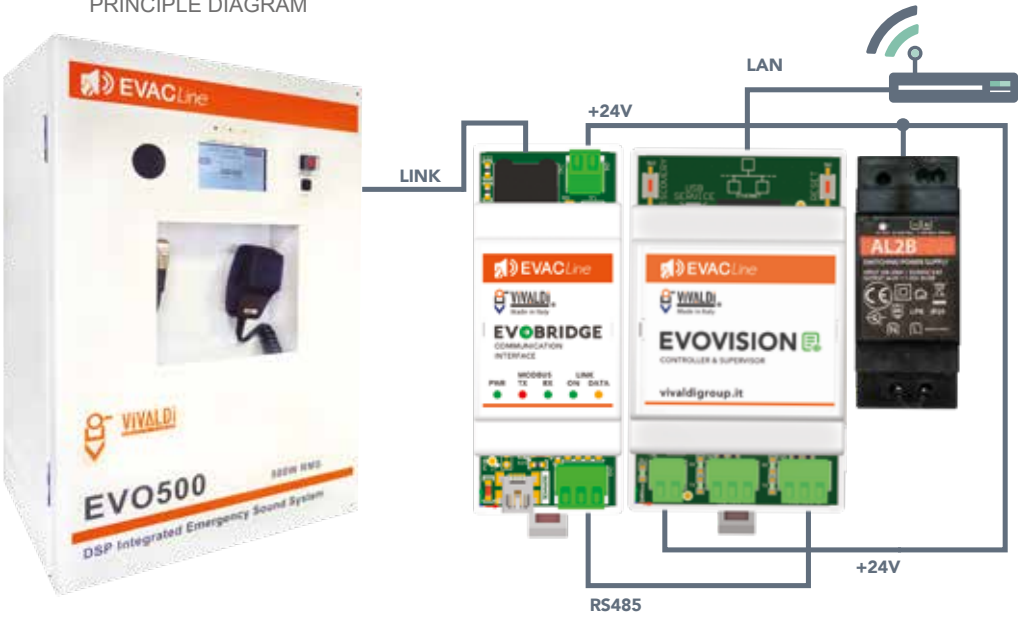
SCHEMA DI PRINCIPIO PRINCIPLE DIAGRAM
