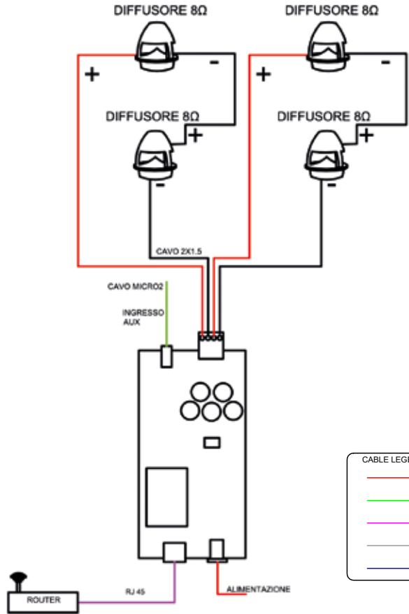
COLLEGAMENTO IN SERIE DI N.4 DIFFUSORI DA GIARDINO
